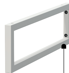
hoekige witte console b 20 x d 450 x h 140 mm
